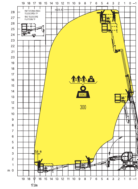
TP O-U telescopisch 3d zwenkbaar werkplatform met 340° rotatie
