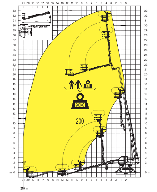
TP O-U telescopisch 3d zwenkbaar werkplatform met 340° rotatie
